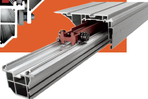
Formátovací vozík s přesným vedením na kalených tyčích
